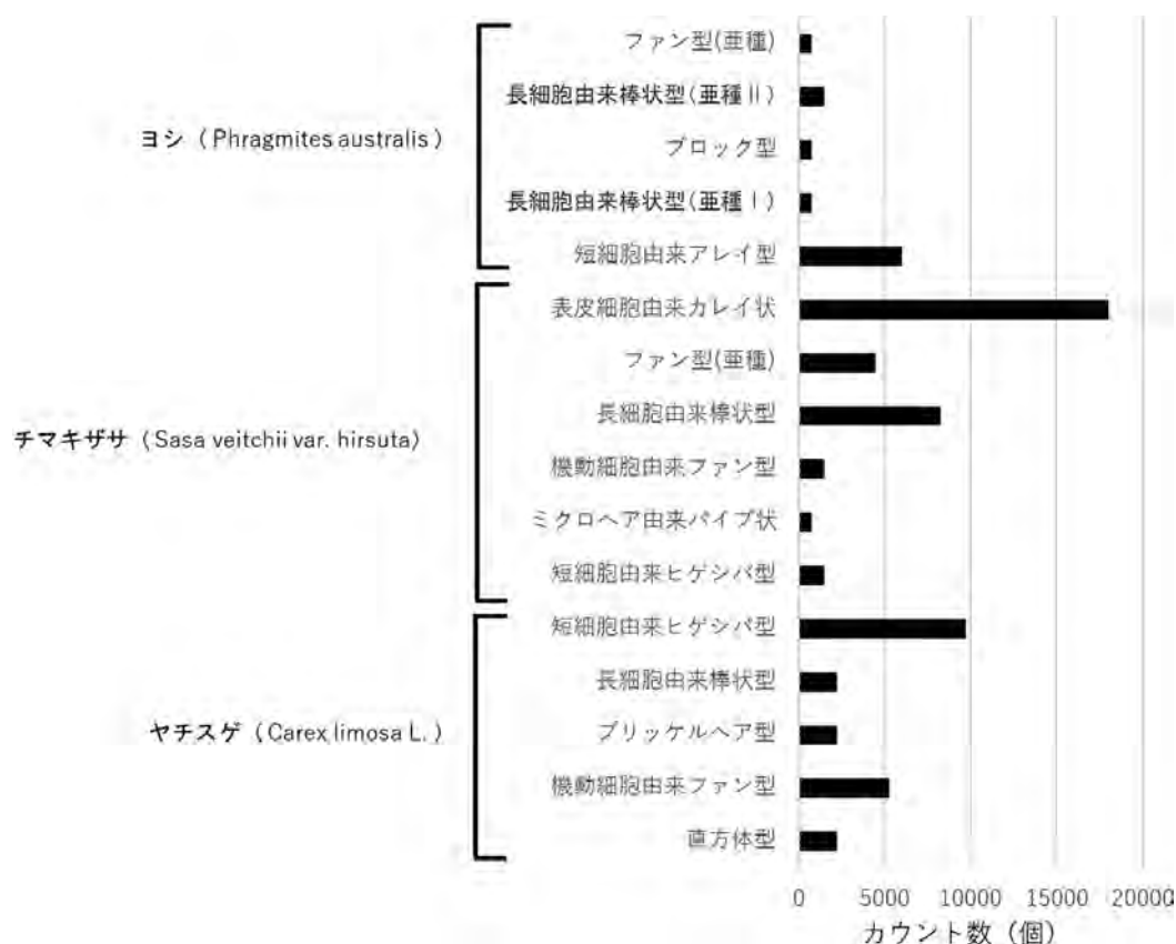
図4 表層堆積物中（15cm）から検出された植物珪酸体組成
