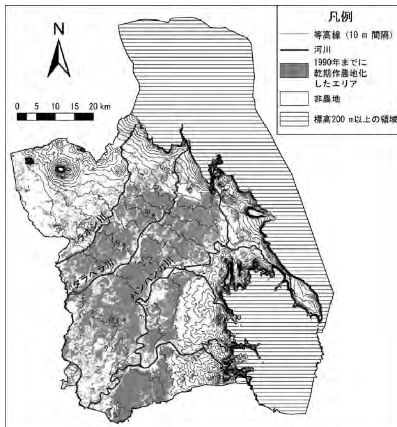
図5 乾期作農地の抽出地域と地形的特徴
